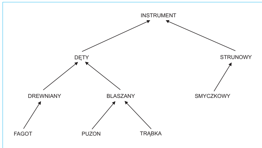
Rysunek 3.17. Przykładowa hierarchia klas z dziedziczeniem pojedynczym
